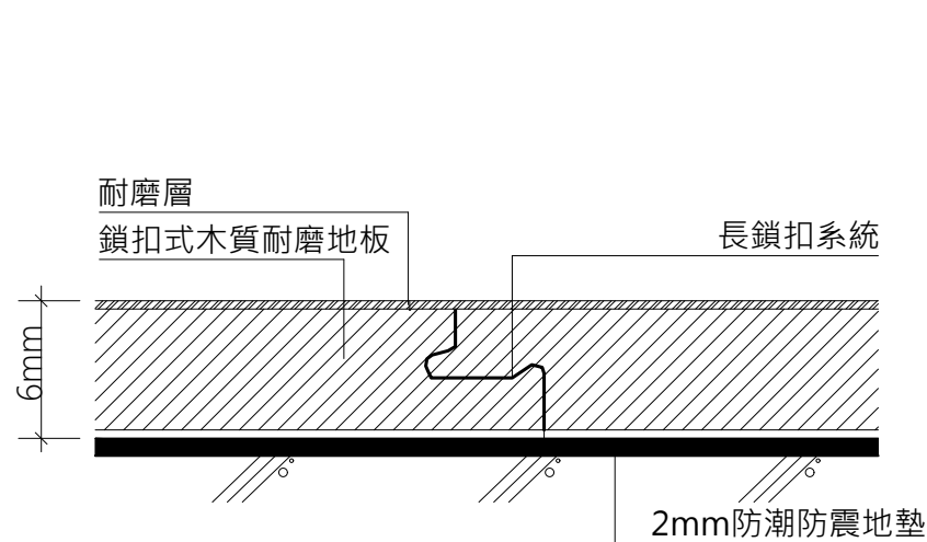
板片接合示意圖
