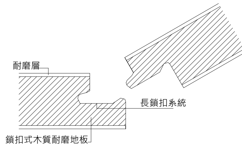
板片接合處大樣示意圖
